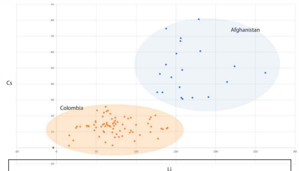
फिगर 5. LA-ICPMS से सूक्ष्म विश्लेषण करने पर हम देख सकते हैं कि कौन सा एमरल्डस कहाँ का है.. बायनरी प्लाट्स प्रक्रिया का इसमें उपयोग किया गया है।
