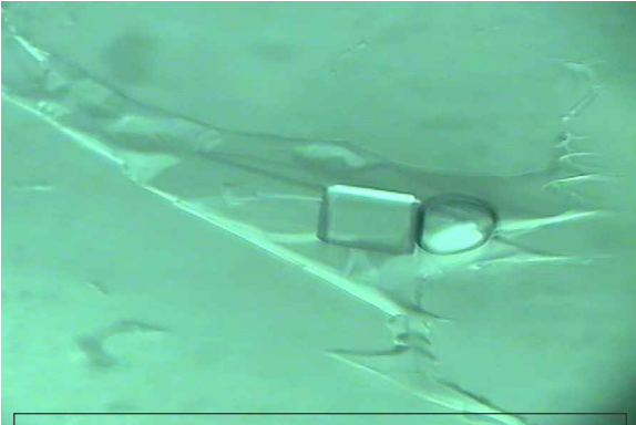
फिगर 4. कोलंबियन एमरल्डस में जैगेड- 3 फेज इनक्लूजन, जिसमें नजर आ रही है फ्लुइड्स फिल्ड कैवैटी, बबल के रूप में ट्रेड गैस और ठोस क्रिस्टल। हालांकि यह सब अफगानी एमरल्डस में भी देखने को मिलता है। फ्लुइड्स फिल्ड कैवैटीज में एकाधिक क्रिस्टल देखने को मिल जाते हैं।
