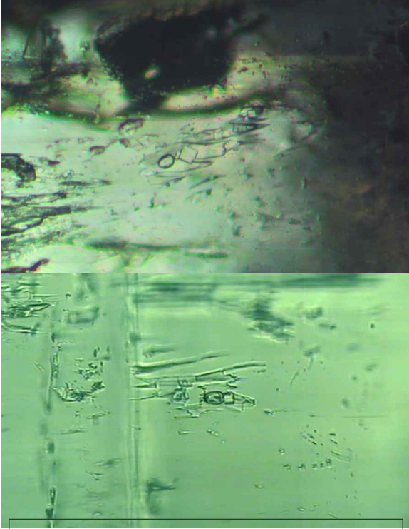
फिगर 3. कोलंबियन एमरल्डस (ऊपर) और अफगानी एमरल्डस(नीचे) का इनक्लूजन सीन। फ्लुइड्स फिल्ड कैवैटीज और जैड परतों से अनुमान लगा सकते हैं। बिना ट्रेस एलीमेंट कैमिस्ट्री के पता लगाना सच में कठिन काम है।
