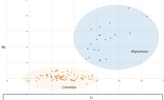
फिगर 6. बायनरी प्लाट्स प्रक्रिया से अफगानी एमरल्डस कैसा होता है, यह सूक्ष्मता से देखा समझा जा सकता है।
