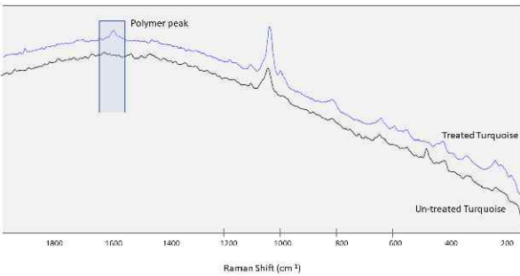
रमन स्पेक्ट्रा प्रक्रिया के दौरान प्राकृतिक (काला निशान) और बहुलक-उपचारित टर्कोइज (नीला ट्रेस)।
