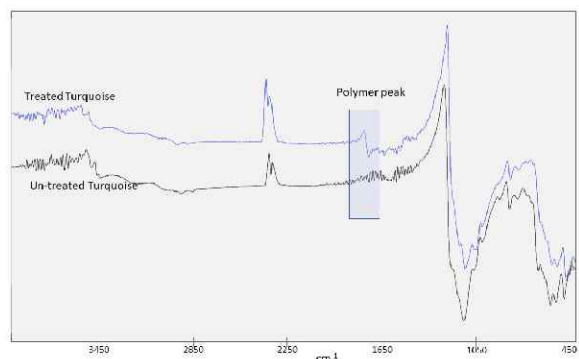
इन्फ्रारेड स्पेक्ट्रा द्वारा प्राकृतिक (ब्लैक ट्रेस) और पॉलीमर-ट्रीटेड टर्कोइज (ब्लू ट्रेस)।
