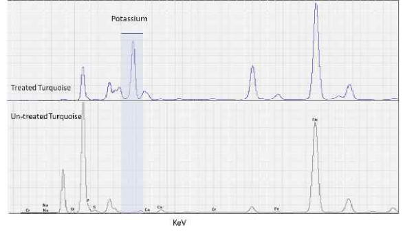
'जैकरी-उपचारित' टर्कोइज (टॉप) पोटेशियम की उच्च सांद्रता प्रदर्शित करता है, जो प्राकृतिक टर्कोइज में अनुपस्थित है।
