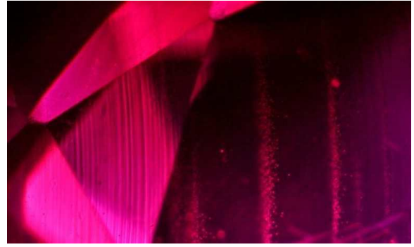
चित्र 4: कलर्ड (घुमावदार) ग्रोथ लाइन्स और बारीक पार्टिकल्स के घुमावदार जोन ने पुष्टि की कि यह 6.20 कैरेट का सैपल वर्नुइल सिंथेटिक रूबी है।
