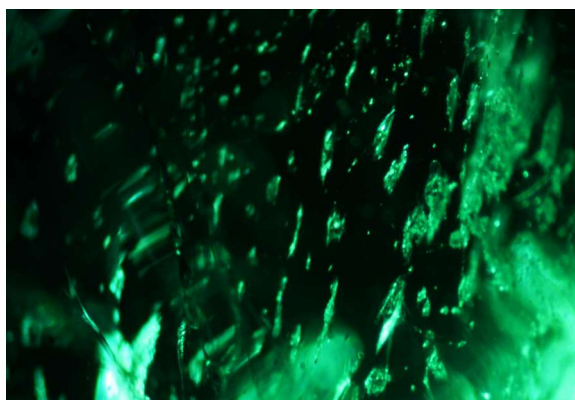
चित्र 4: ब्राज़ील, इथियोपिया और ज़ाम्बिया से आने वाले पत्तों में २-फेज़ इनक्लूजन के साथ सफेदी लिए धुंधली फिल्म आम तौर पर देखी जा सकती है।
